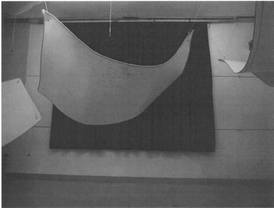
Abbildung B.1. Prüfanordnung im Hallraum (Ansicht).
